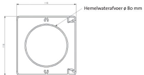
Doorsnede van standaard staander van bovenaf gezien:
