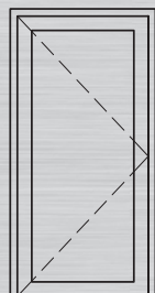
AANZICHT ENKELE DEUR
