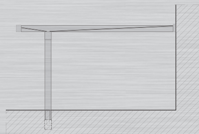
DOORSNEDE ULTRALINE CLASSIC
